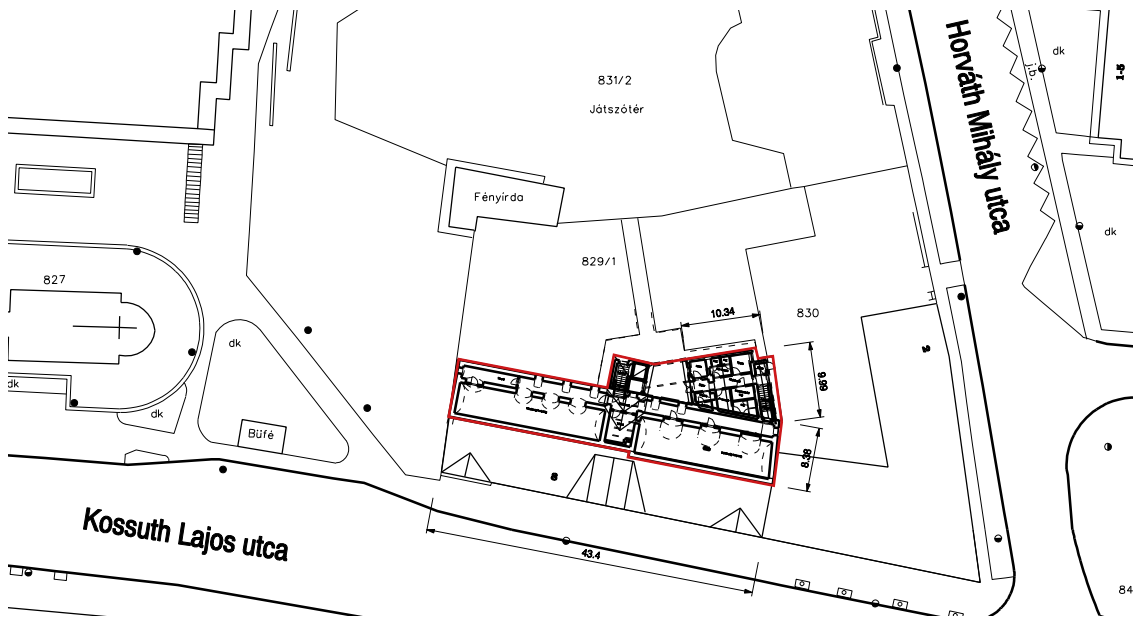
15. A Diák Pince elhelyezkedése és körvonal rajza a Kossuth L. u. 8. sz. ház alatt
