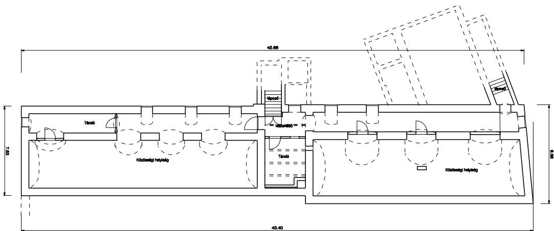
16. A Diák Pince két nagytermének vázrajza
