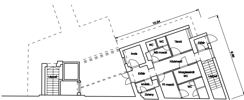
17. A Diák Pince földszinti (vizesblokk) alaprajza
